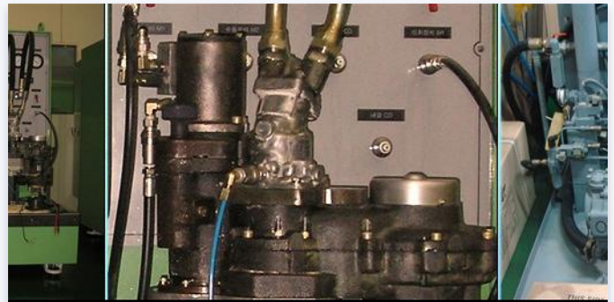
기어/구동장치 시험장비 K1/K1A1 선회장치 시험장비
