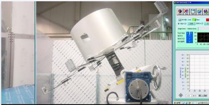
기타 시험장비 인공위성안테나 시험장비
